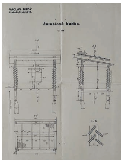
Plánek žaluziové budky pro plánovanou meteorologickou stanici
